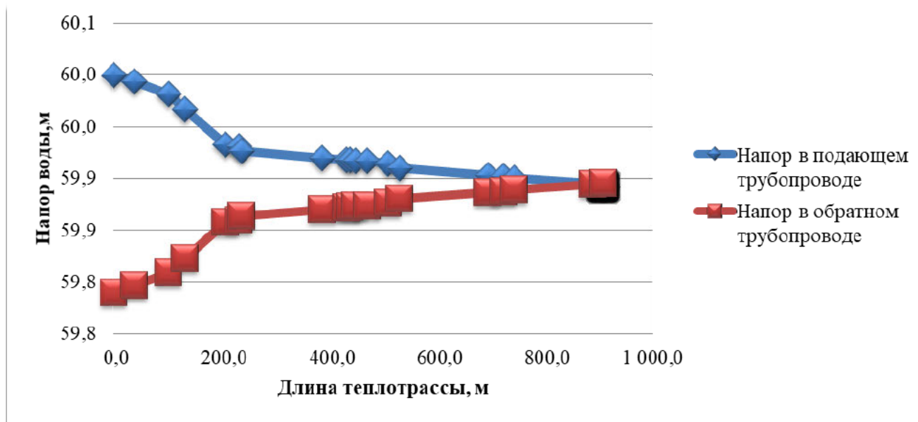
Рисунок 2.3 – Пьезометрический график тепловой сети котельной п. Новопокровка по магистральному выводу
