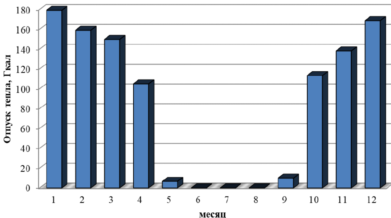
Рисунок 1.2 – Оптимальный температурный график отпуски тепловой энергии для котельной п. Новопокровка
